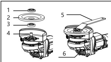
1. Buitenflens 4. As 2. Schijf 5. Borgmoersleutel 3. Binnenflens 6. Asvergrendeling
