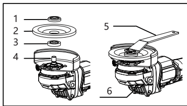
1. Flangia esterna 4. Mandrino 2. Disco 5. Brugola 3. Flangia interna 6. Blocco del mandrino
