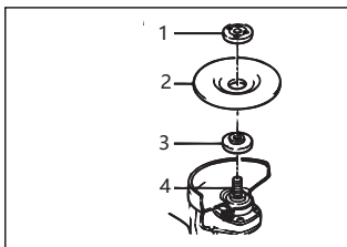
1. Brida exterior 2. Rueda central presionada 3. Brida interior 4. Husillo de conducción
