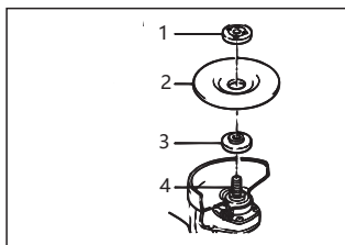
1. Flasque extérieur 2. Rondelle concave 3. Flasque intérieur 4. Arbre d'entraînement
